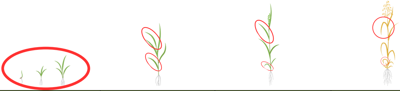
TILLERING
